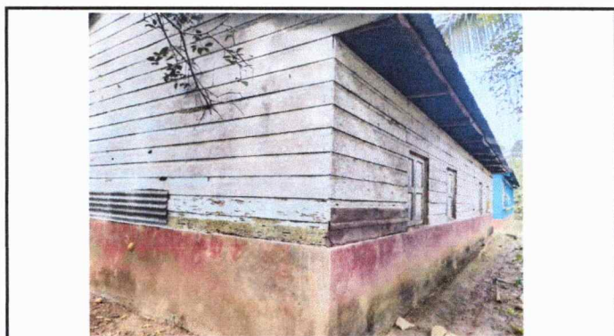
Foto 4: Se observa las paredes exteriores bastante deterioradas por la humedad debido a su exposición a las inclemencias del tiempo.
